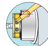
COMO REGULAR MOTOR AUTOMÁTICO PARA PERSIANA INTEGRADA E CORTINA
