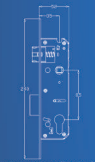
Máquina de porta de giro com 52mm de profundidade (M35G-POR/VE)
