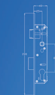
Máquina de porta de giro com 40mm de profundidade (M25G-POR/VE)
