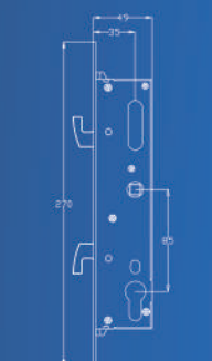
Máquina de porta de correr com 40mm de profundidade (M25C-POR/VE)
