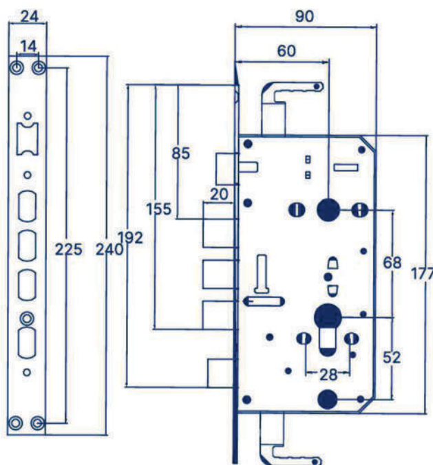
Máquina padrão Spring lock 24mm
