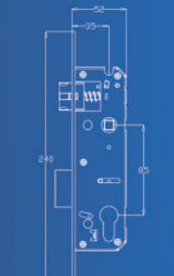
Máquina de porta de giro com 52mm de profundidade (M35G-POR/VE)
