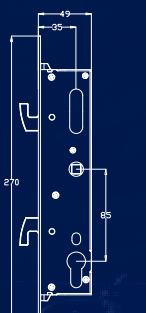
Máquina de porta de correr com 49mm de profundidade (M35C-POR/VIE)
